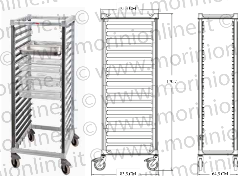
203076 - CARRELLO PORTATERGLIE/BACINELLE CM 73X43,8 H 170,7 PER 18 TEGLIE GN 2/1 O 36 TEGLIE GN 1/1 H 6,5 ■ Specifiche - Struttura in poliuretano, nylon rinforzato e polipropilene rinforzato, ogni guida ha una portata massima di 36 Kg, con una capacità massima di carico per il carrello pari a 340 Kg. Il carrello è in grado di ospitare teglie appena uscite dal forno con una temperatura pari o inferiore a 200°C
